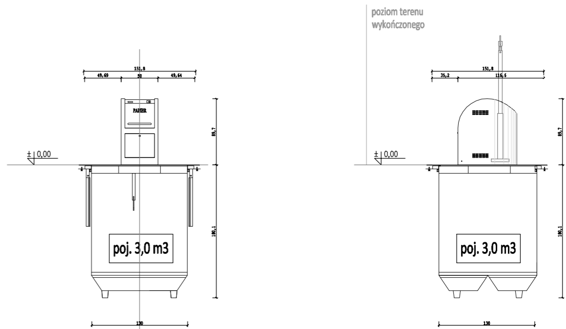
PRZEKRÓJ A-A
